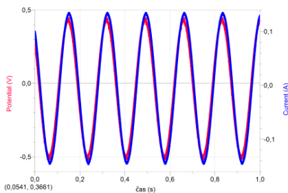
Obr. 3 Frekvence zdroje 5 Hz, fázové posunutí prakticky nulové
