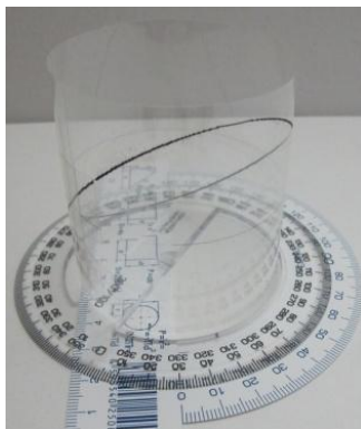
Obr. 5 Lissajousova křivka poměr frekvencí 1:1 pro fázový posun 30^\circ
