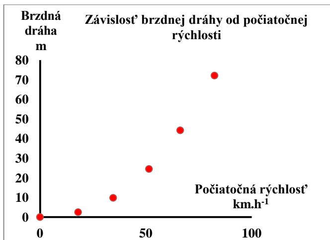
Obr. 3 Grafické spracovanie výsledkov urania, závislosť brzdnjej dráhy auta od jeho počiatočnej rýchlosti
