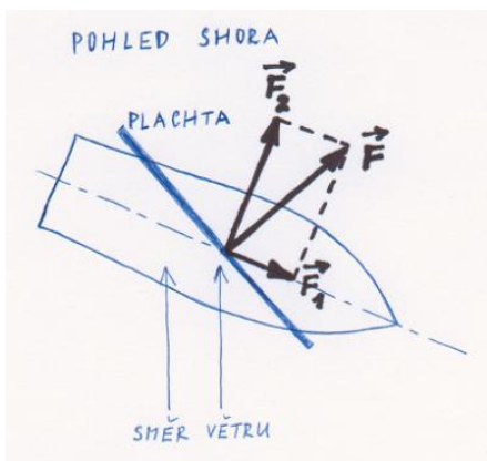
Obr. 3 Náčrtek plachetnice s působícími silami
