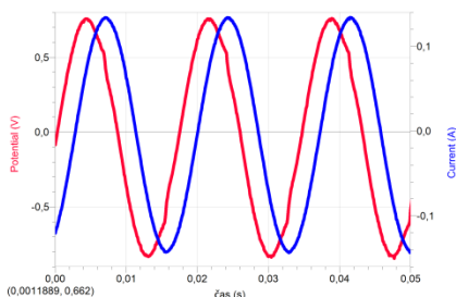
Obr. 4 Frekvence zdroje 50 Hz, fázové posunutí zhruba 45^\circ
