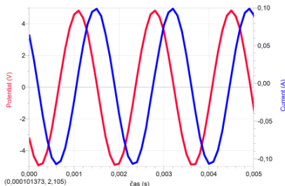
Obr. 5 Frekvence zdroje 500 Hz, fázové posunutí téměř 90^\circ
