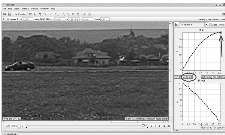
Obr. 2 Zo závislosti polohy automobilu od času zistíme jeho brzdnú dráhu, v našom prípade približne 25 m
