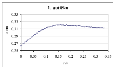
Grafy 3 a 4 Závislost polohy na čase přijíždějícího a původně stojícího autíčka
