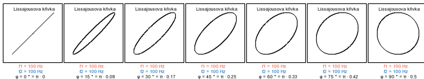
Obr. 1 Lissajousovy obrazce v poměru frekvencí 1:1, a změnou fáze po 15^\circ
