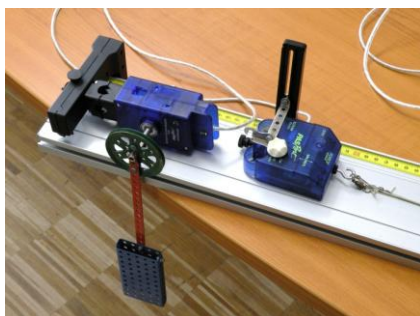
Obr. 2 Senzor rotace (zde jako úhloměř) a senzor síly, umístěné na dráze simulující nakloněnou rovinu
