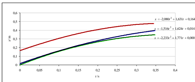
Graf 2 Smykové tření
