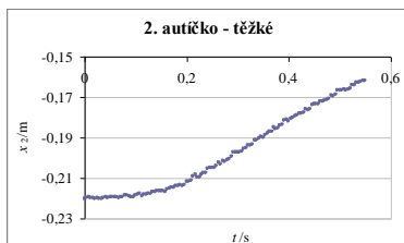
Grafy 5 a 6: Závislost polohy na čase přijíždějícího lehkého a původně stojícího těžkého autíčka
