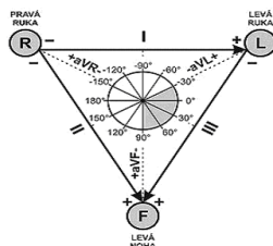
Obr. 2 Eithovenův trojúhelník rozmístění elektrod
