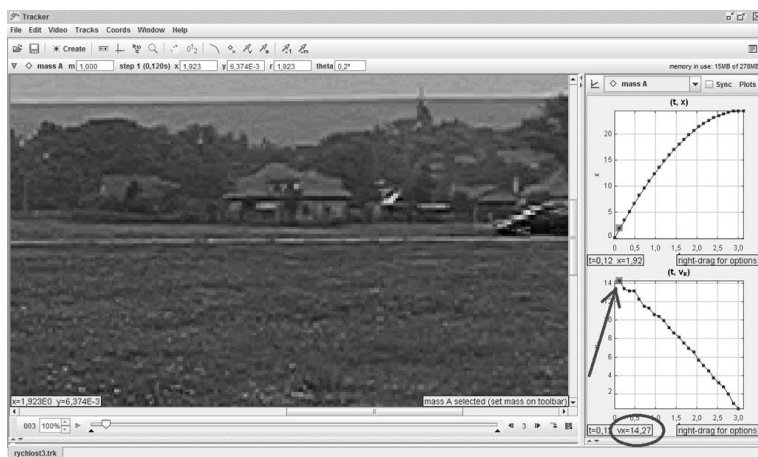
Obr. 1 Zo závislosti rýchlosti automobilu od času zistíme jeho počiatočnú rýchlosť, v našom prípade je počiatočná rýchlosť automobilu približne 14 \text{ m}\cdot\text{s}^{-1}
